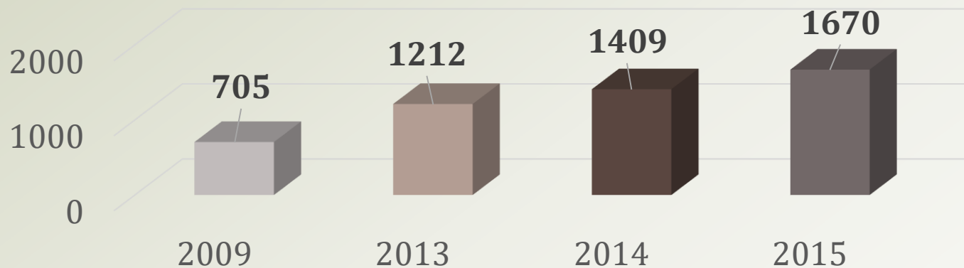
Число операций
