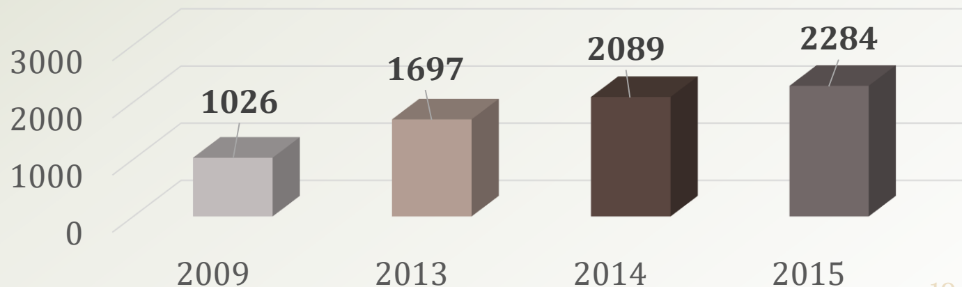
Число операций
